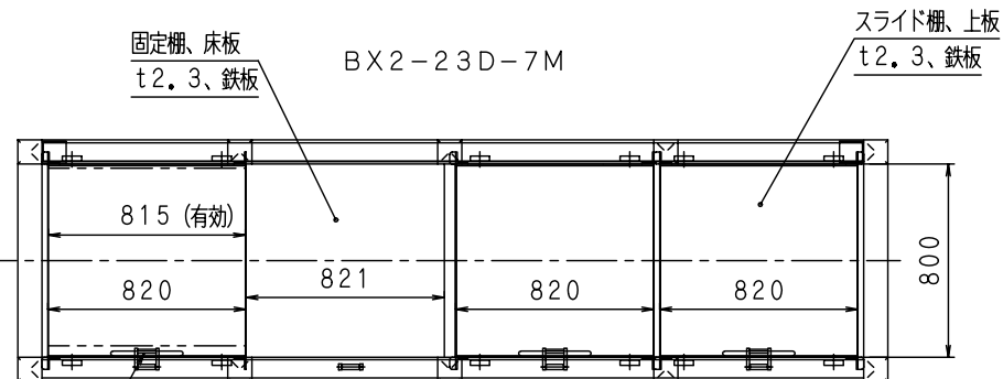
上面図
