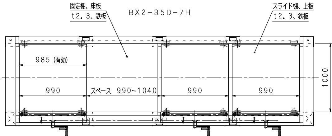
上面図
