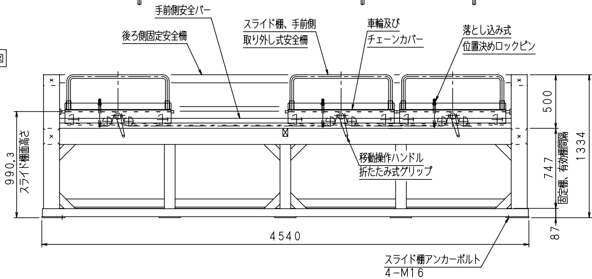
側面図
