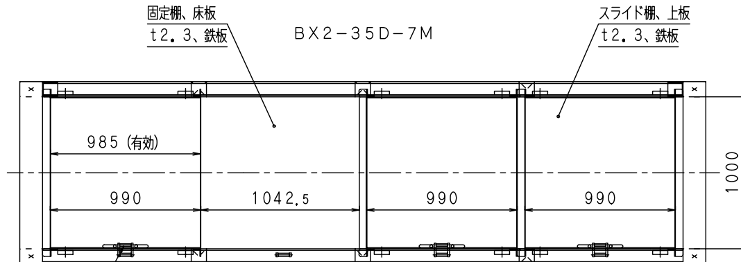
上面図
