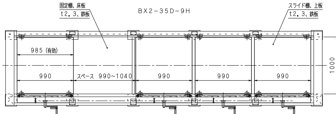
上面図
