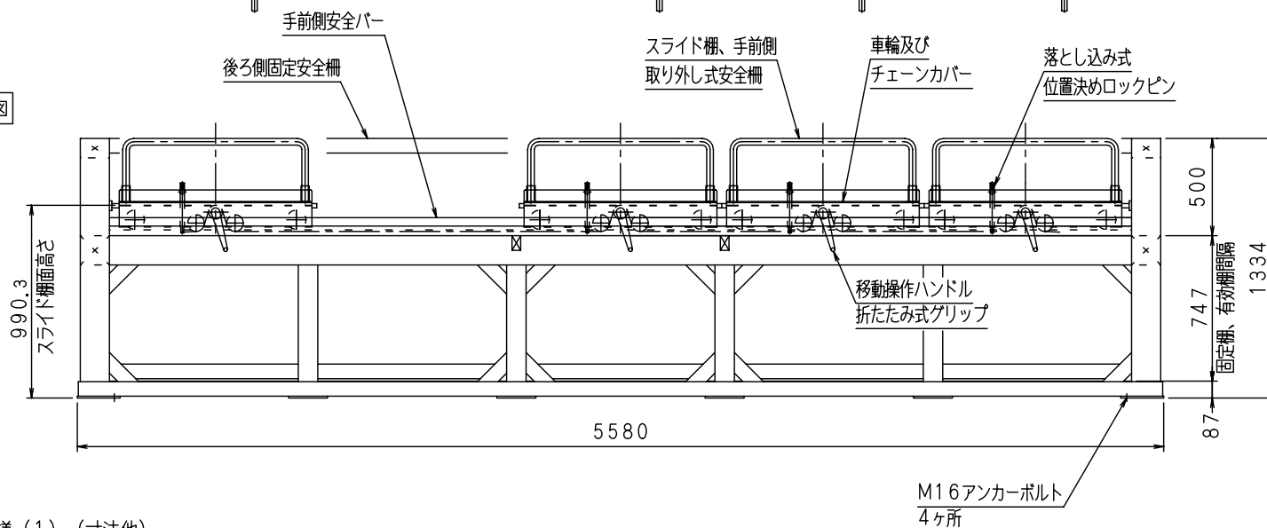
側面図
