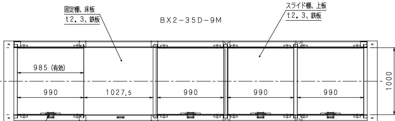
上面図
