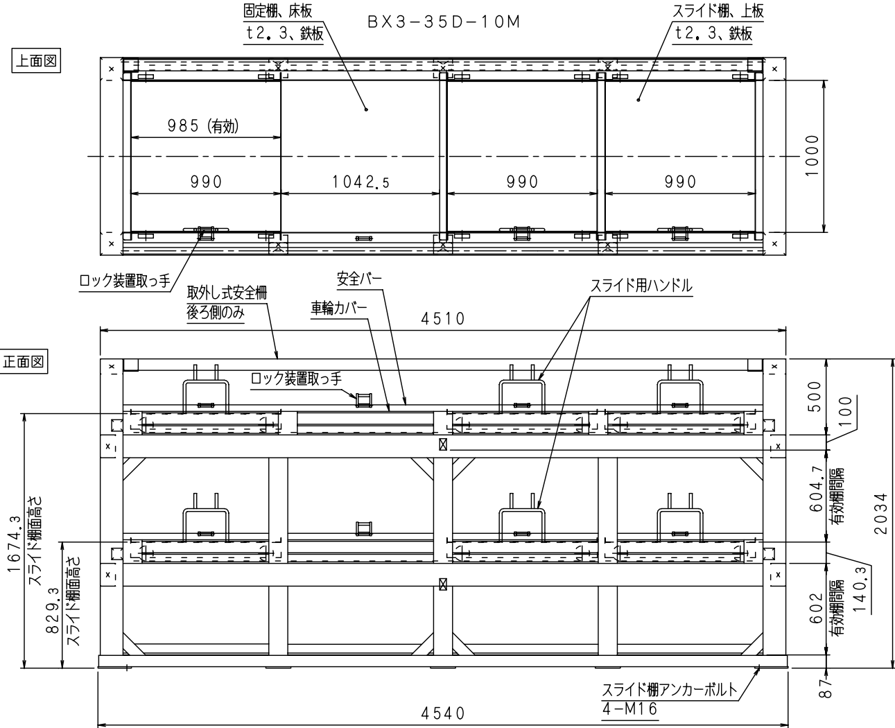
仕様(1) (寸法他)
