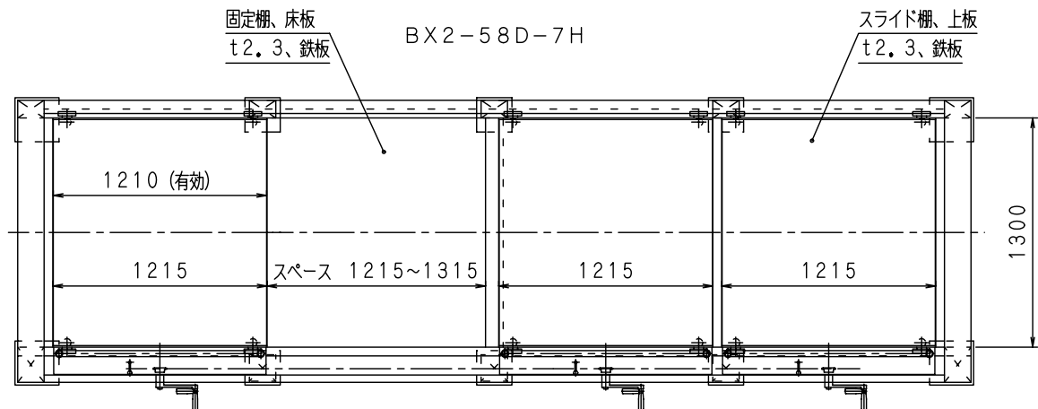
上面図
