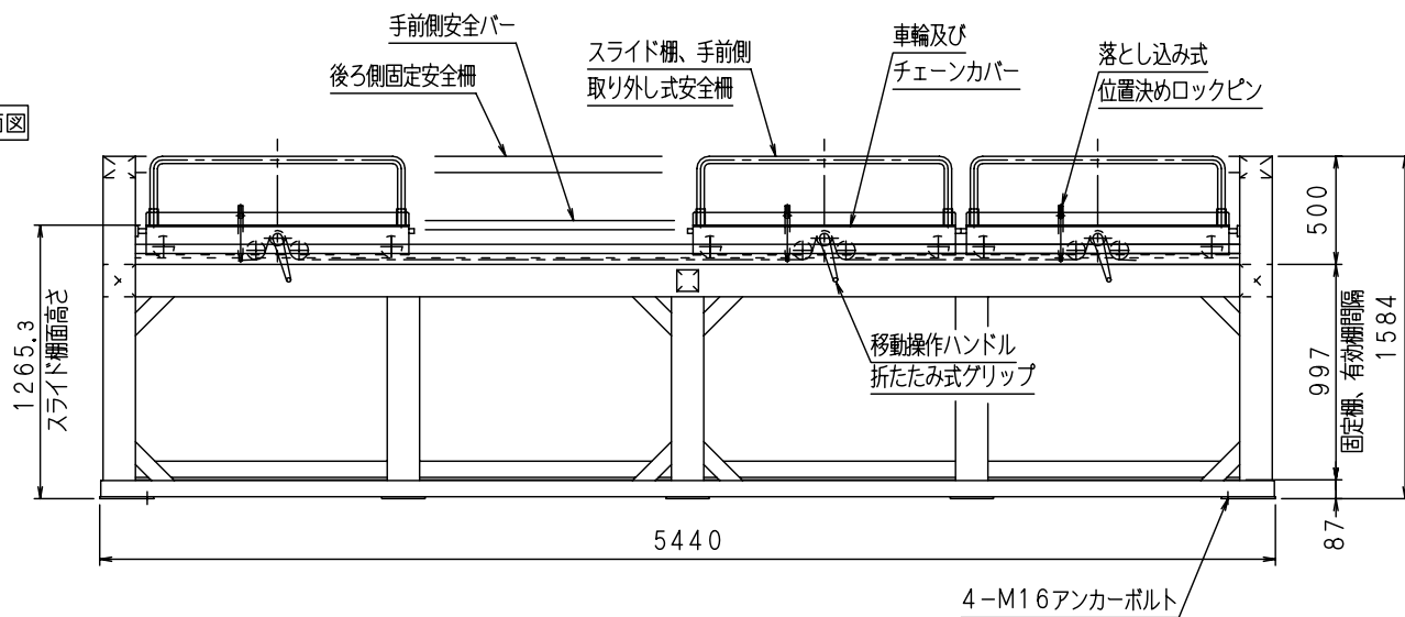
側面図
