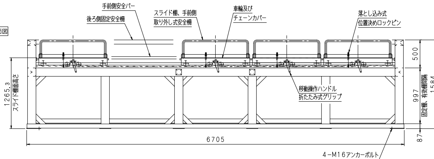
仕様 (1) (寸法他)
