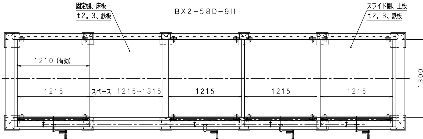
上面図
