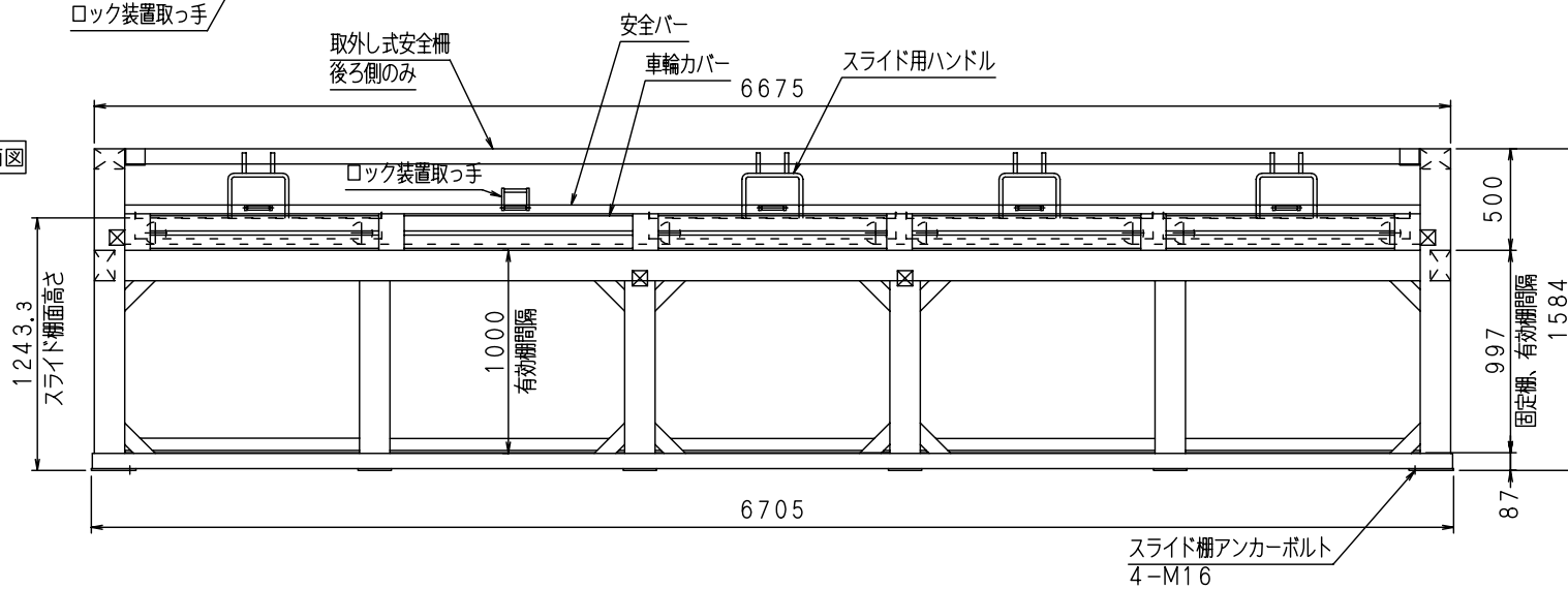
仕様 (1) (寸法他)
