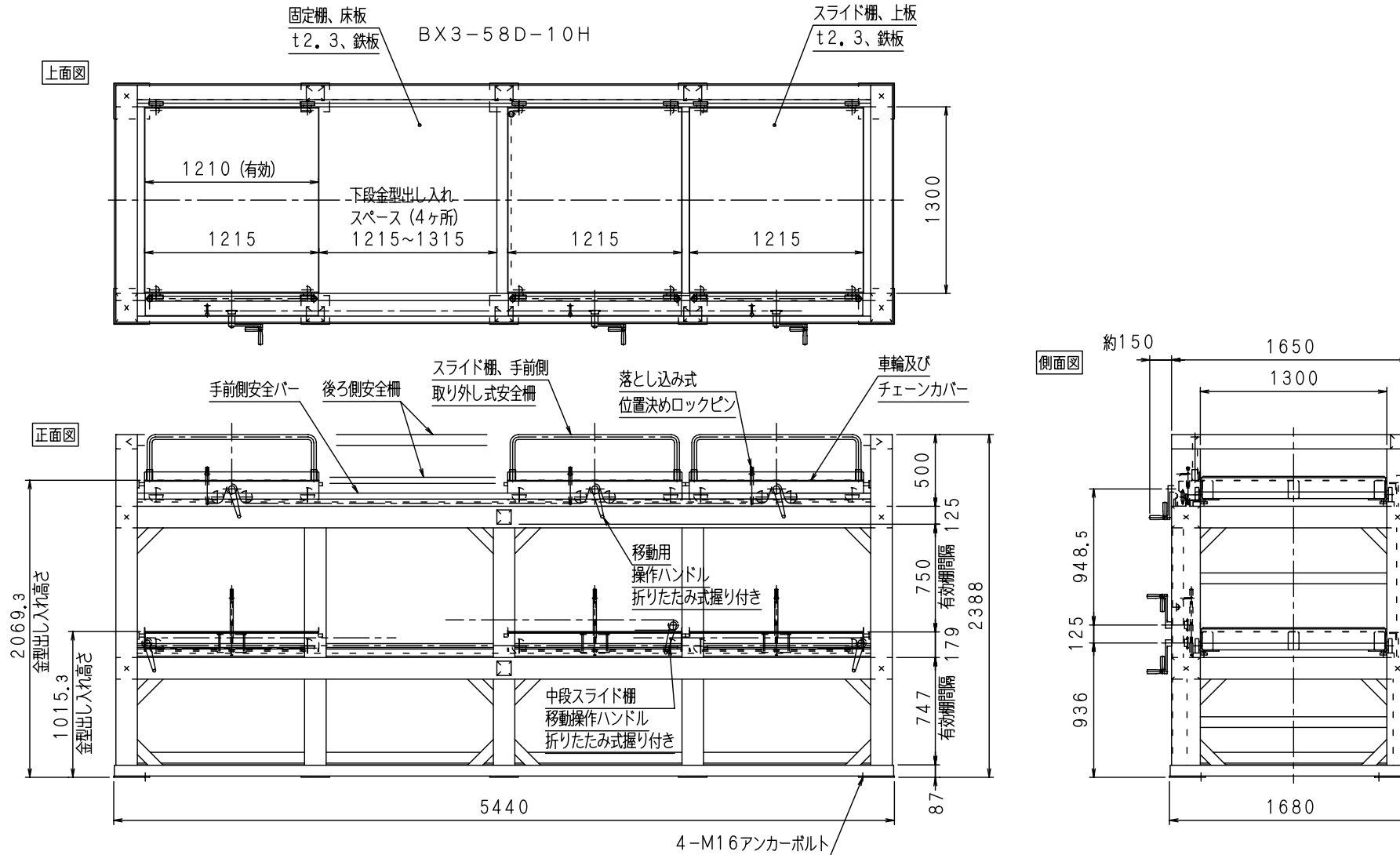
仕様 (1) (寸法他)
