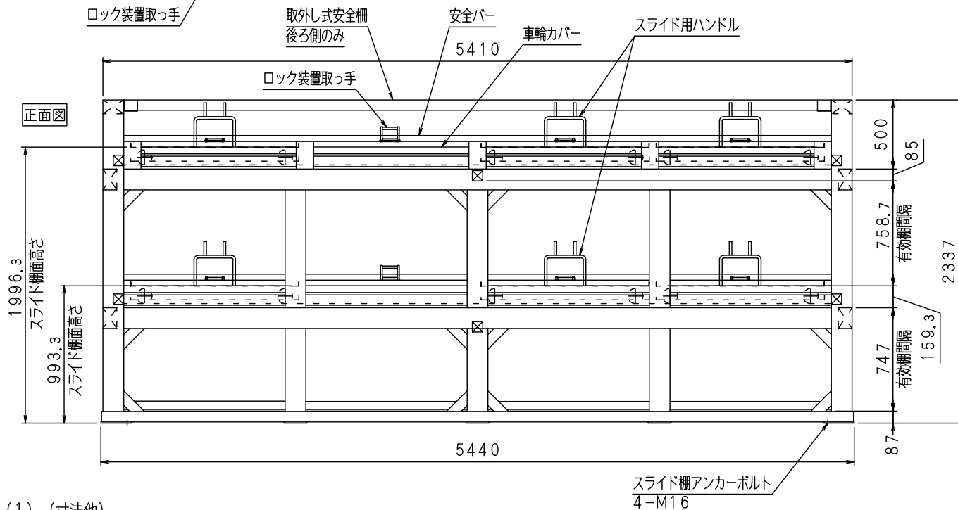
仕様 (1) (寸法他)
