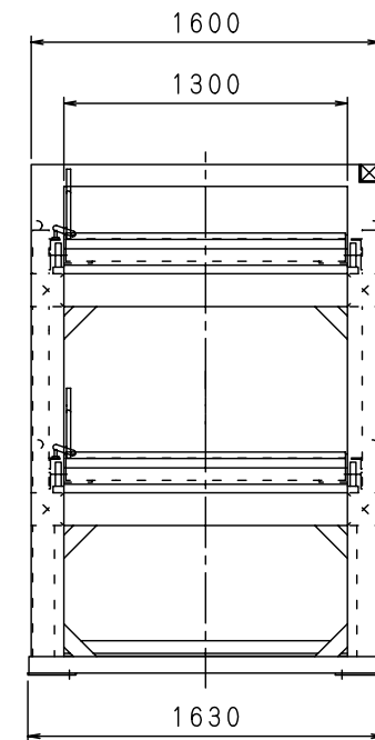
側面図
