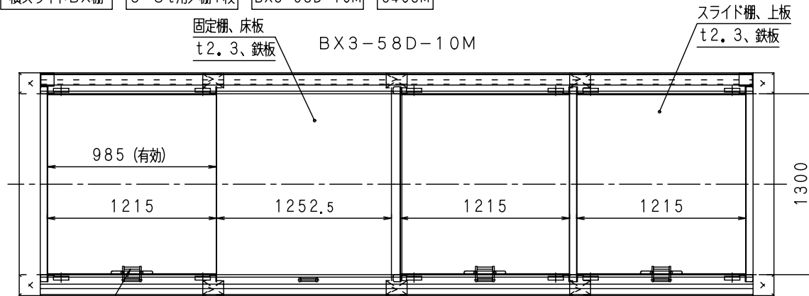
上面図
