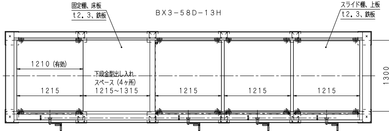
上面図
