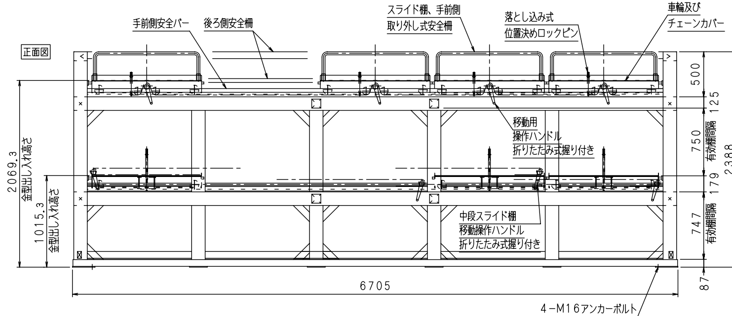
仕様 (1) (寸法他)
