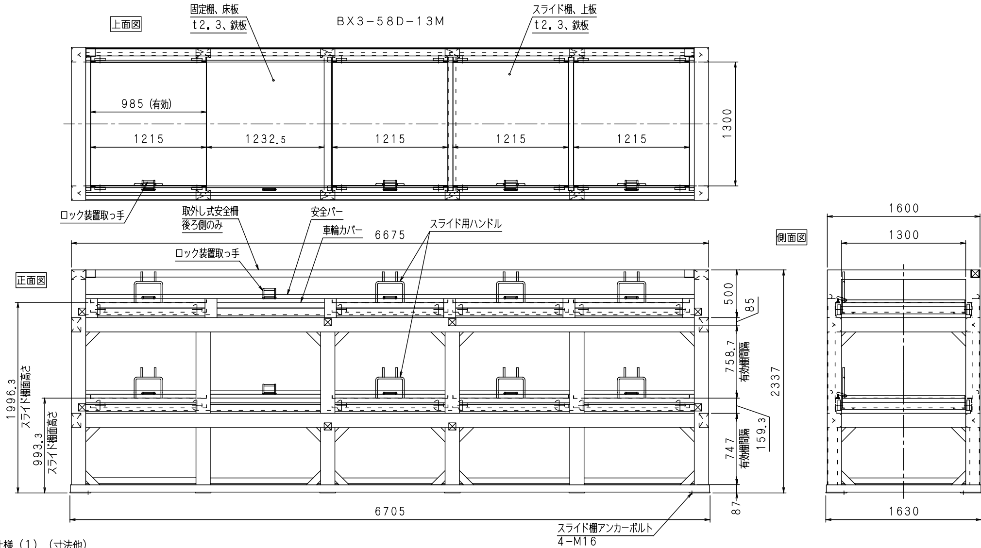
仕様 (1) (寸法他)
