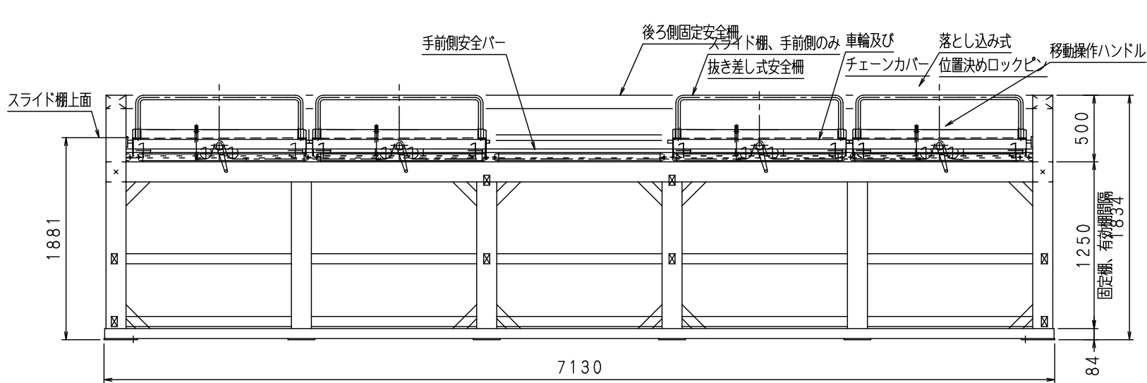
仕様 (1) (寸法他)
