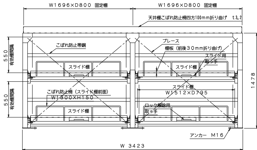
正面図
