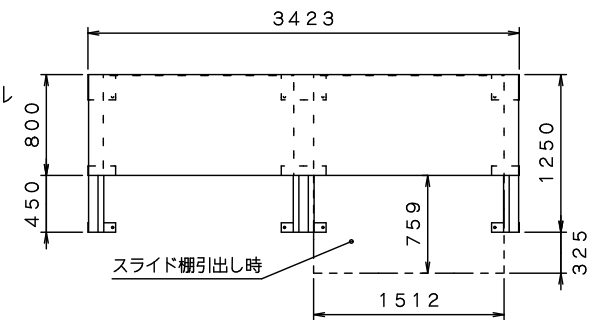
上面図
