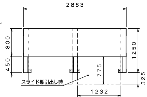
上面図
