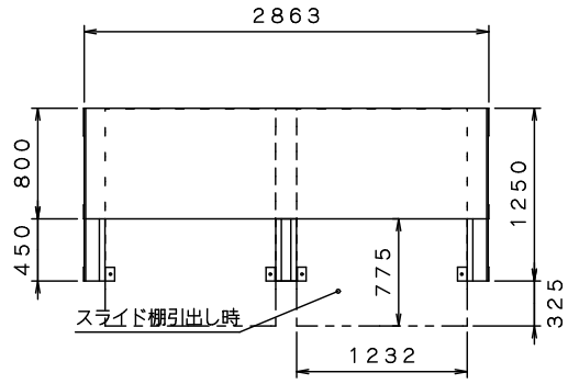
上面図
