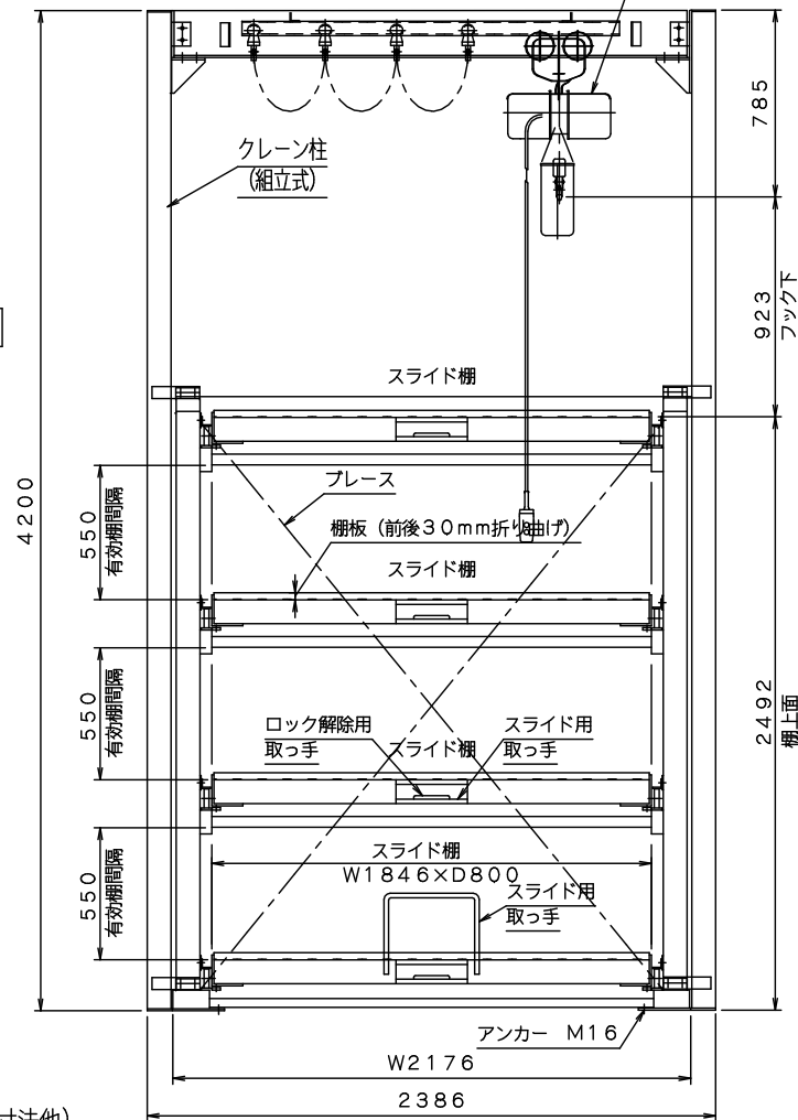
仕様 (1) (寸法他)
