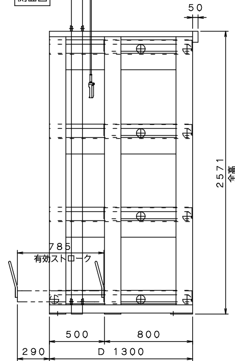
側面図
