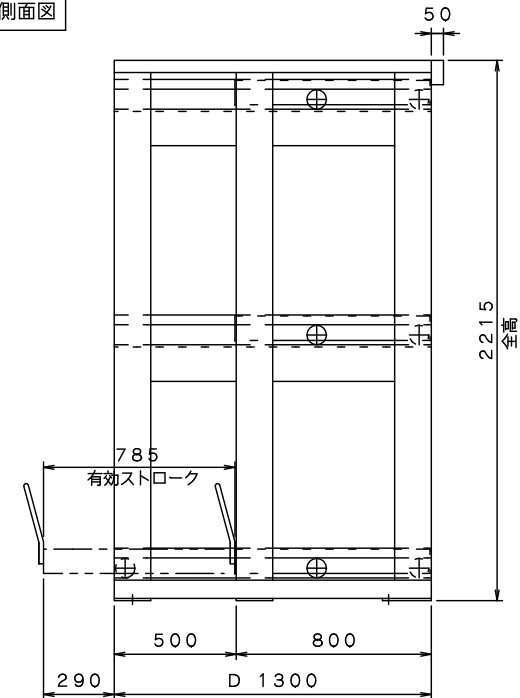
側面図
