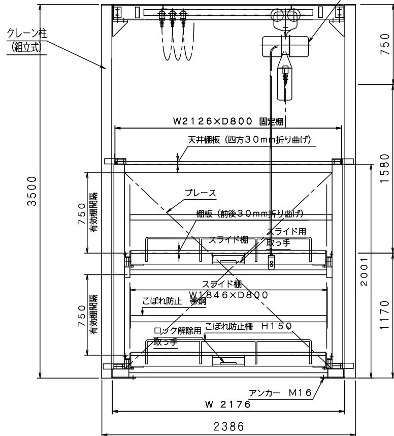
仕様 (1) (寸法他)
