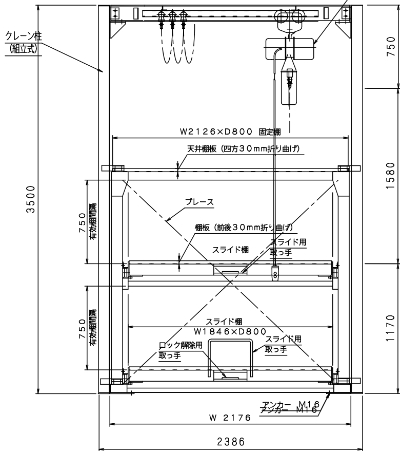
仕様 (1) (寸法他)
