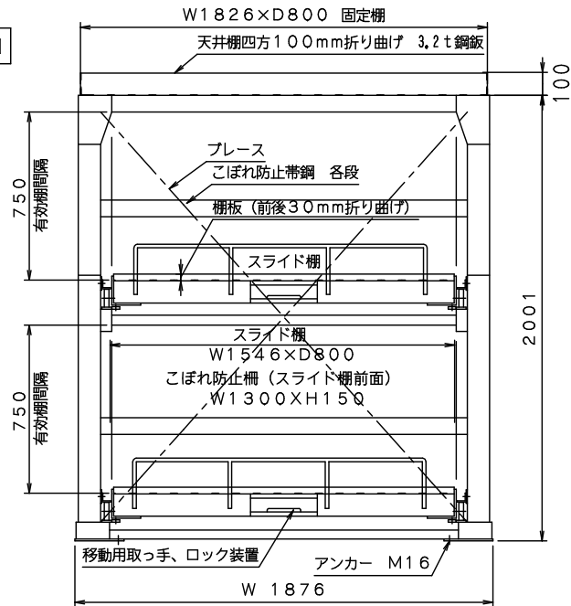
正面図
