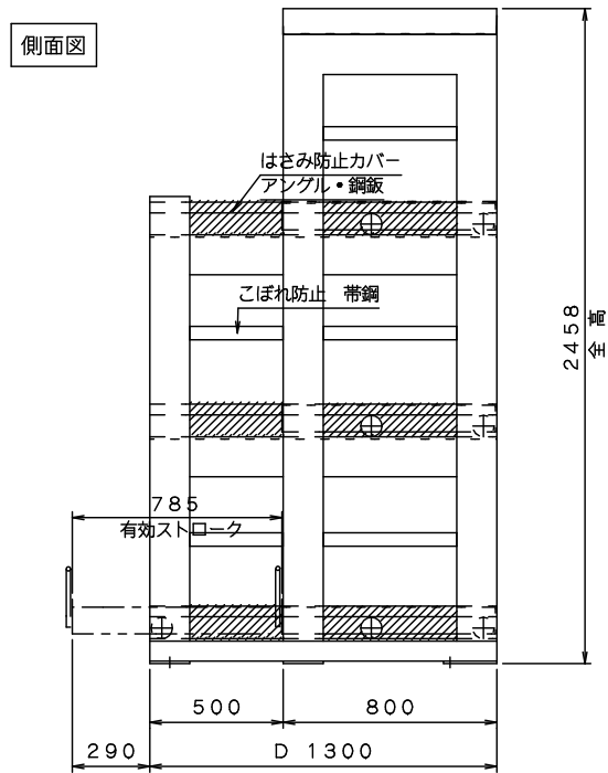
■ 単列 (S) : GSR-4 (15) A フルスライド式
