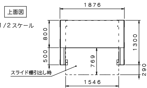
■ 単列 (S) : GSR-4 (15) A フルスライド式
