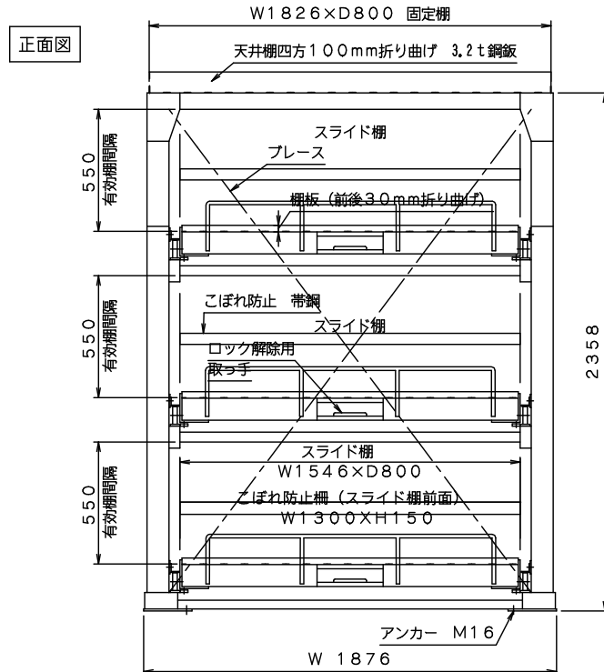
■ 単列 (S) : GSR-4 (15) A フルスライド式
