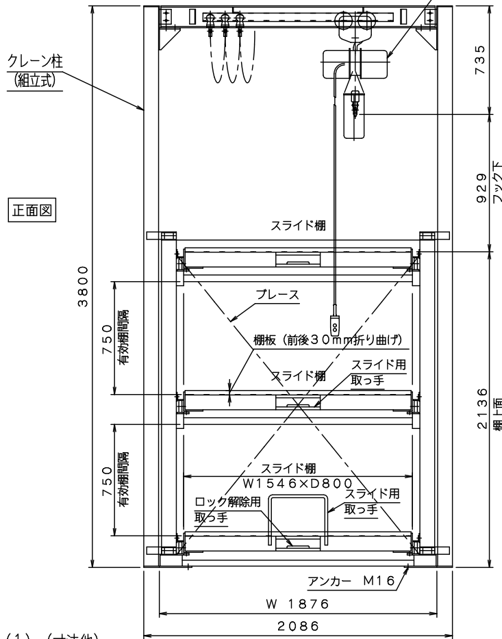
仕様 (1) (寸法他)
