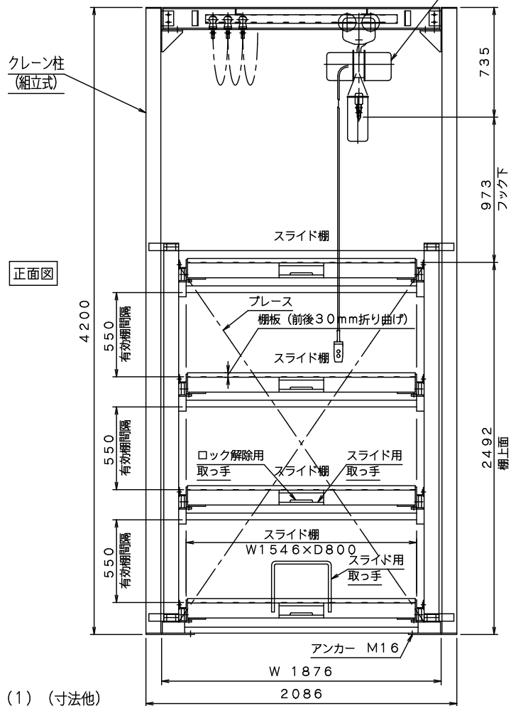
仕様 (1) (寸法他)
