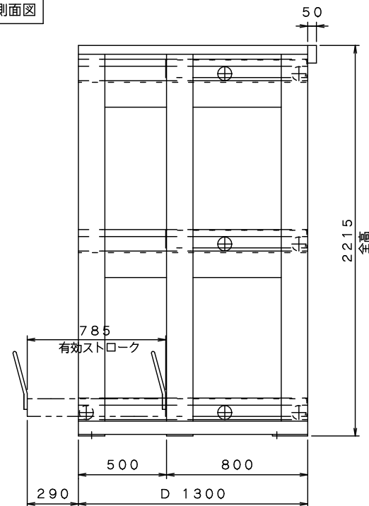
側面図
