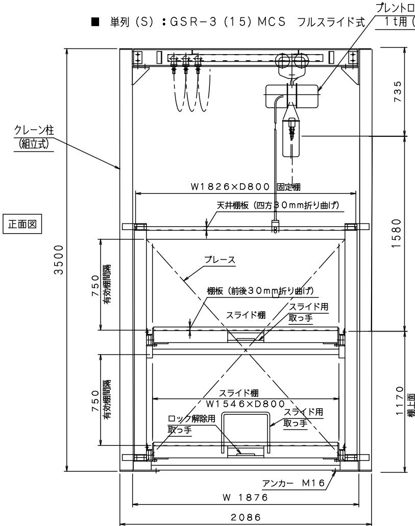
仕様 (1) (寸法他)
