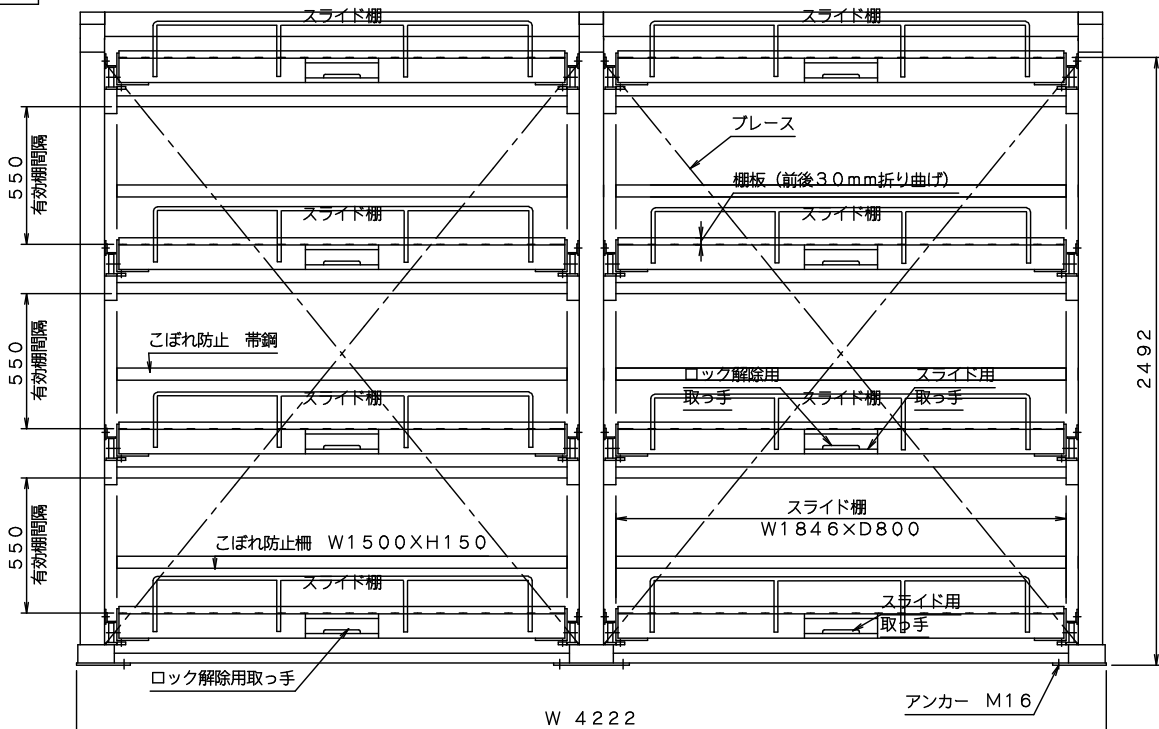
仕様(1) (寸法他)
