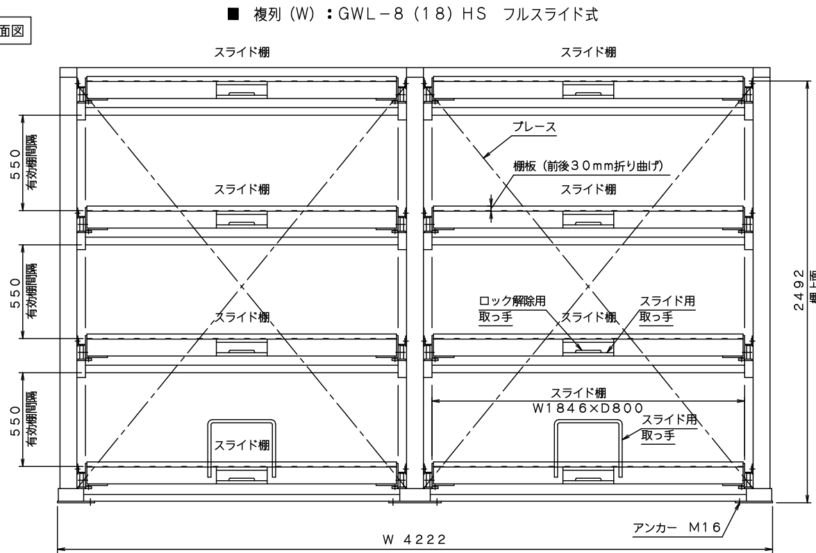
仕様 (1) (寸法他)
