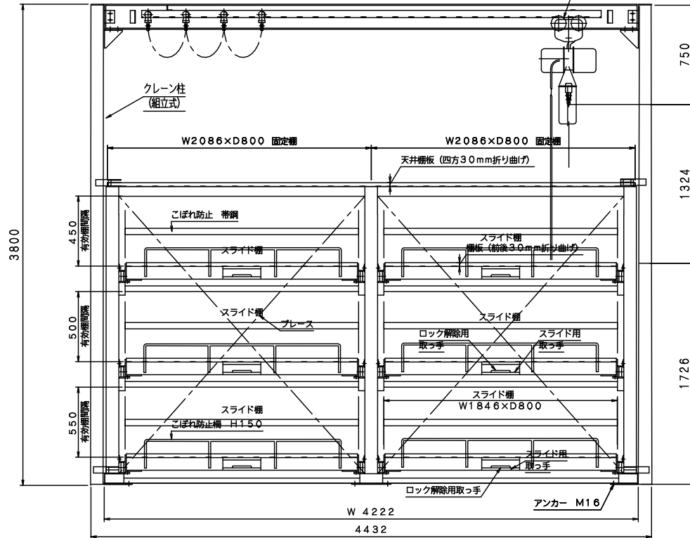
正面図
