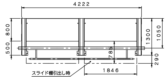
上面図 1/2スケール
