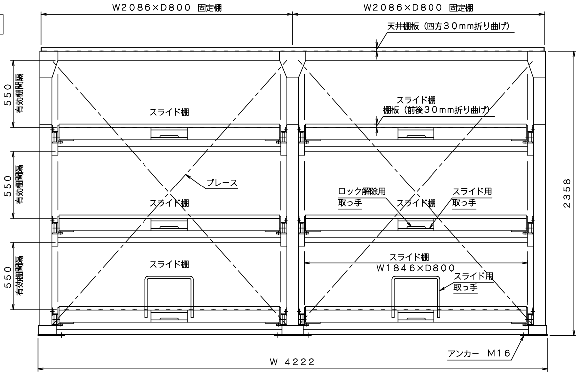
正面図
