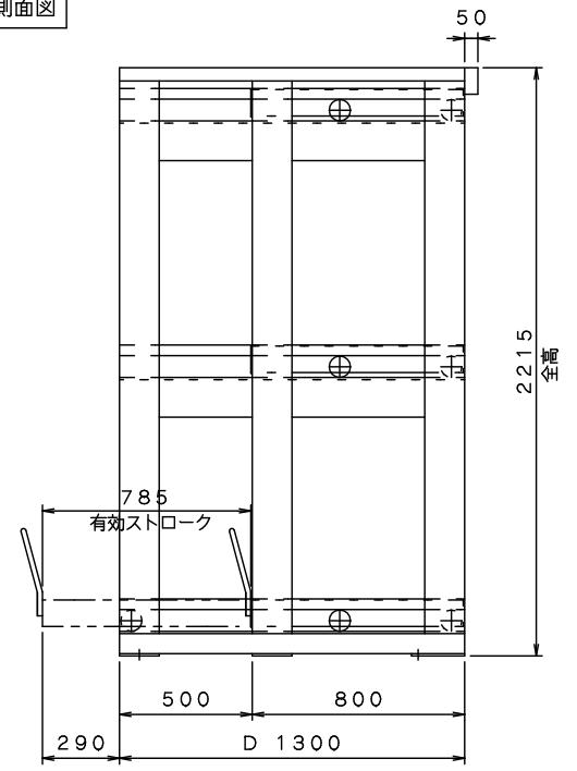
側面図
