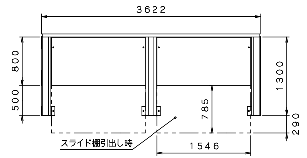
上面図 1/2スケール
