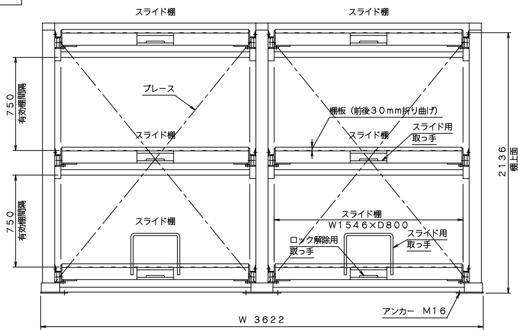
正面図
