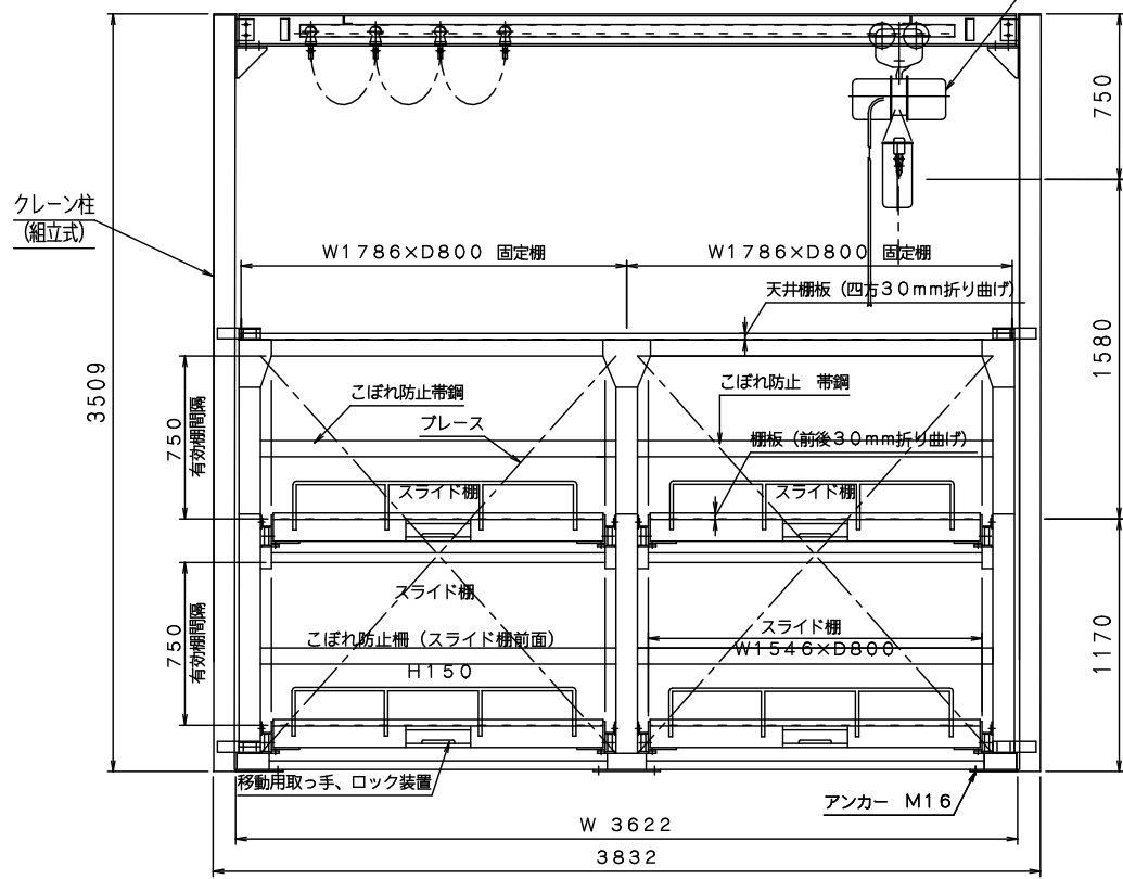
正面図
