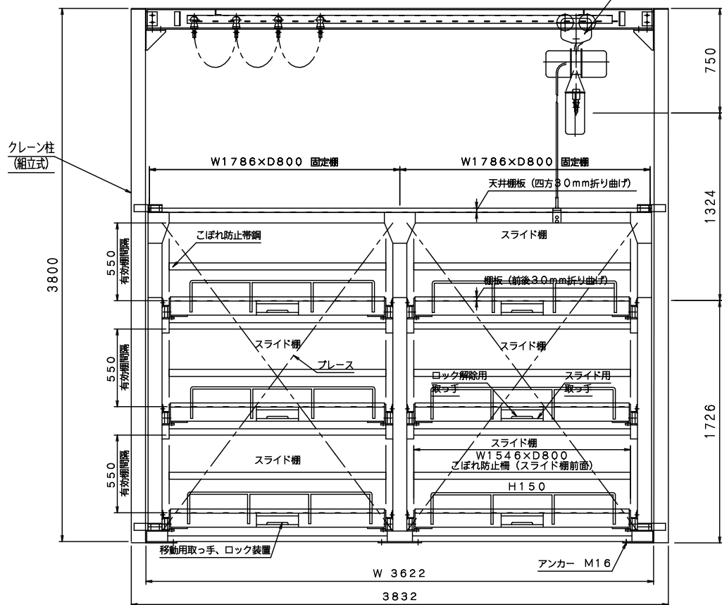
正面図
