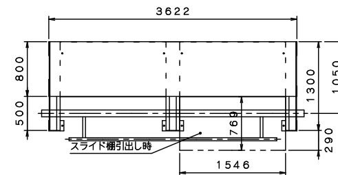
上面図
