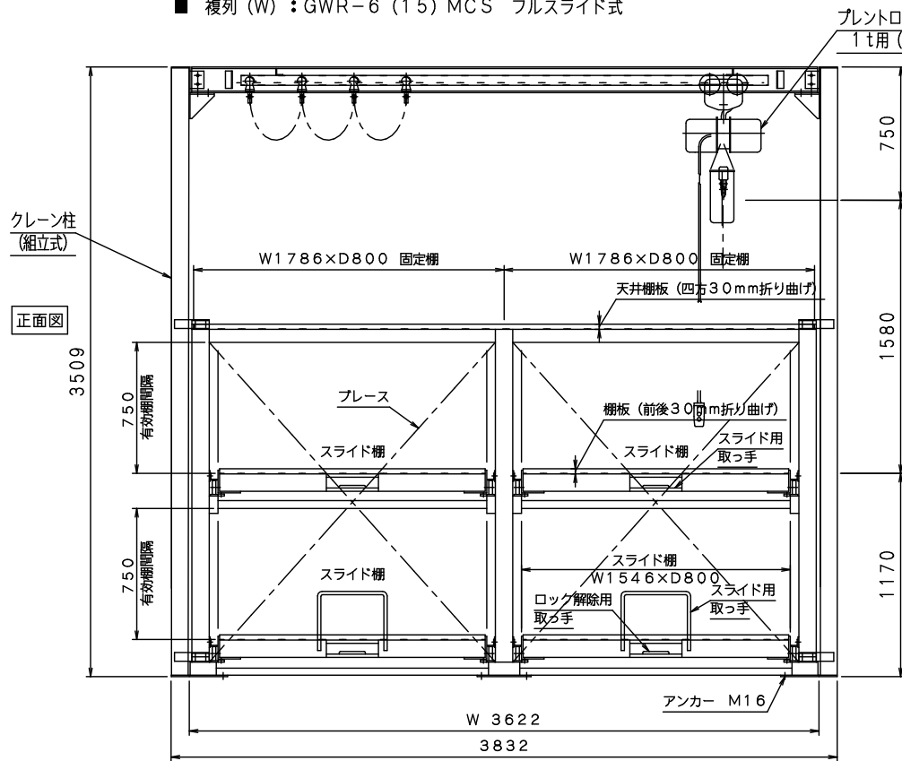
仕様 (1) (寸法他)
