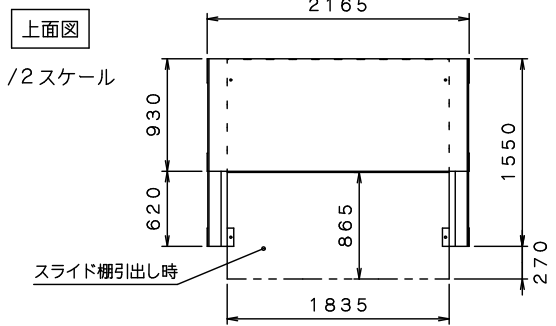
■ 単列 (S) : KSL-3 (18) Aフルスライド式
