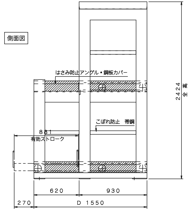
■ 単列 (S) : KSL-3 (18) Aフルスライド式
