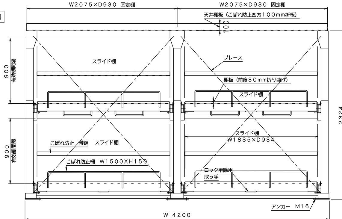
仕様 (1) (寸法他)
