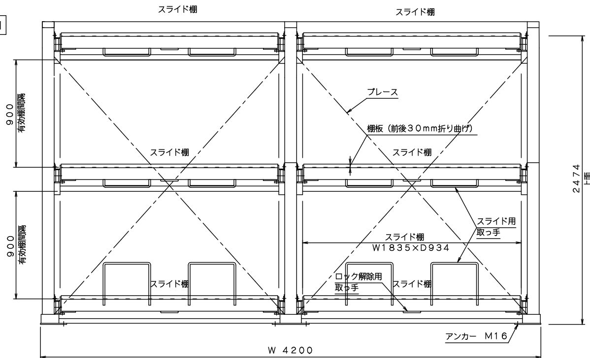
仕様 (1) (寸法他)
