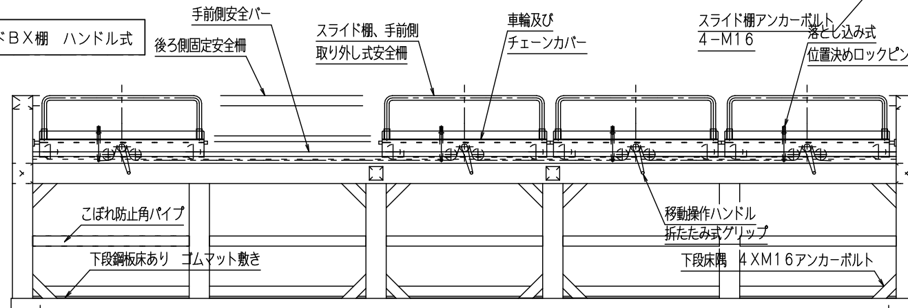
正面図
