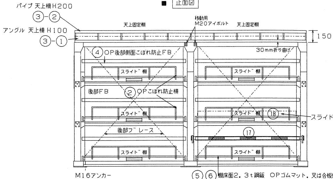
正面図
