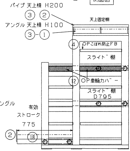
側面図
