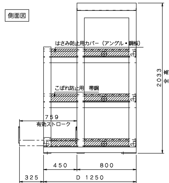
■ 単列 (S) : PSL-4 (18) Aフルスライド式
