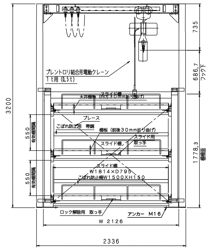
正面図 ■ 単列 (S) : PSL-3 (18) HAフルスライド式
