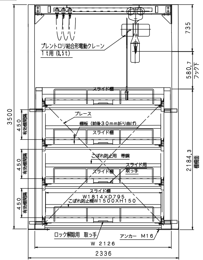
正面図 ■ 単列 (S) : PSL-4 (18) HMCA フルスライド式
