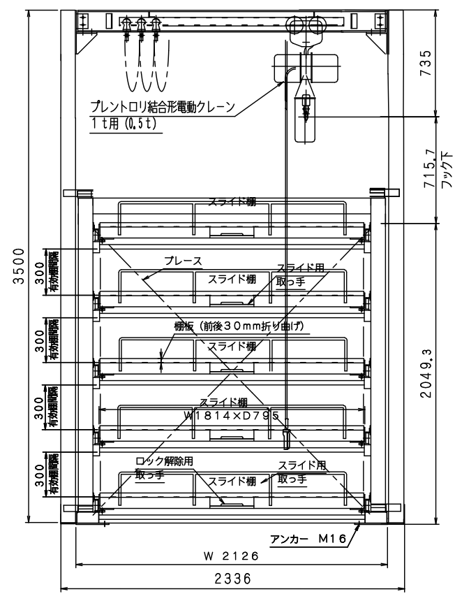
仕様 (2) (寸法他)
