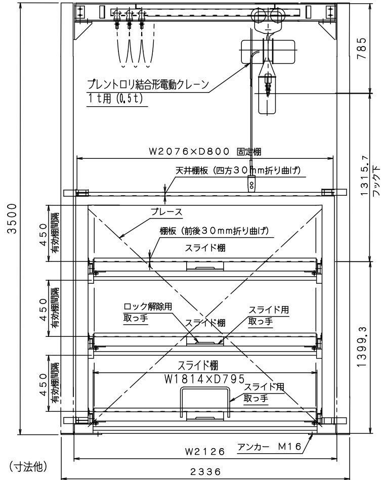
正面図
