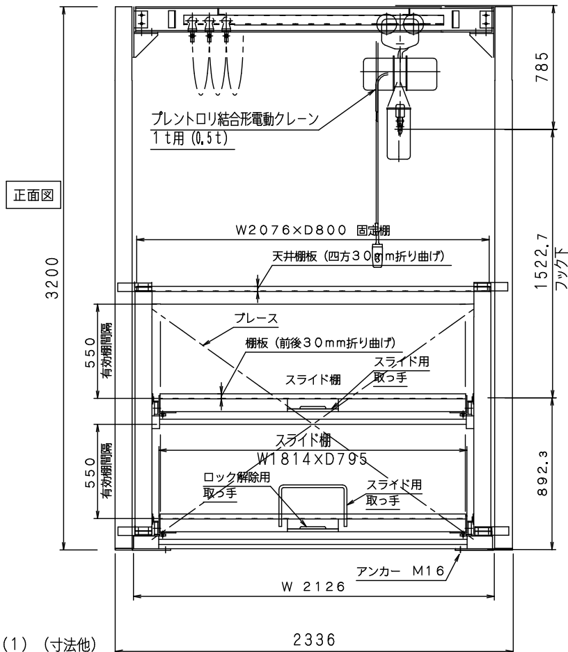
仕様 (1) (寸法他)
