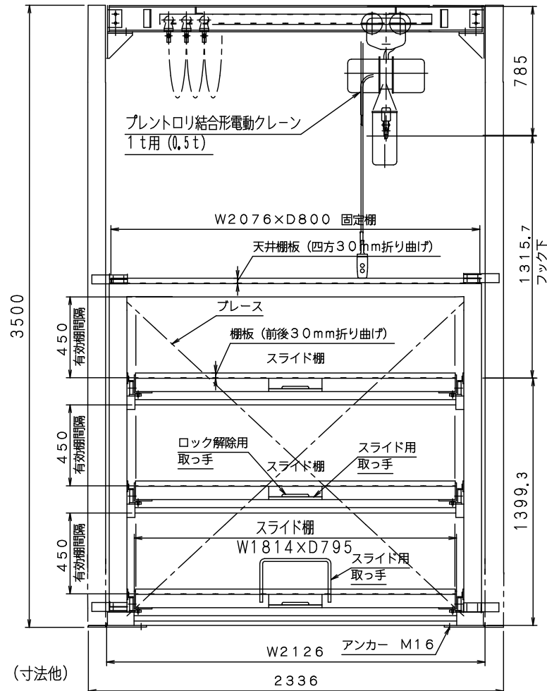
正面図
