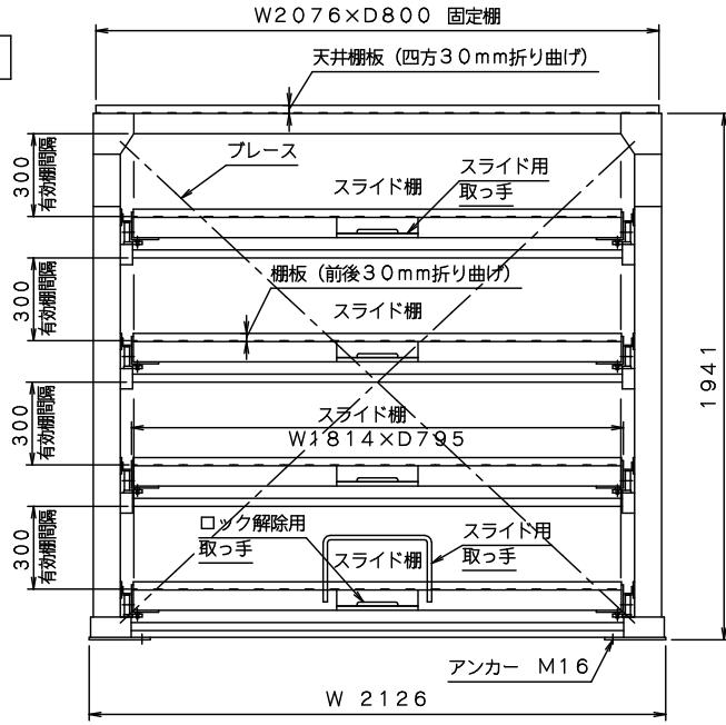
正面図
