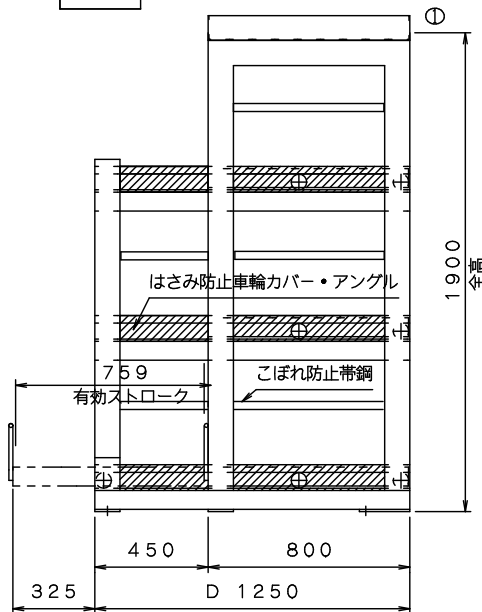
側面図
